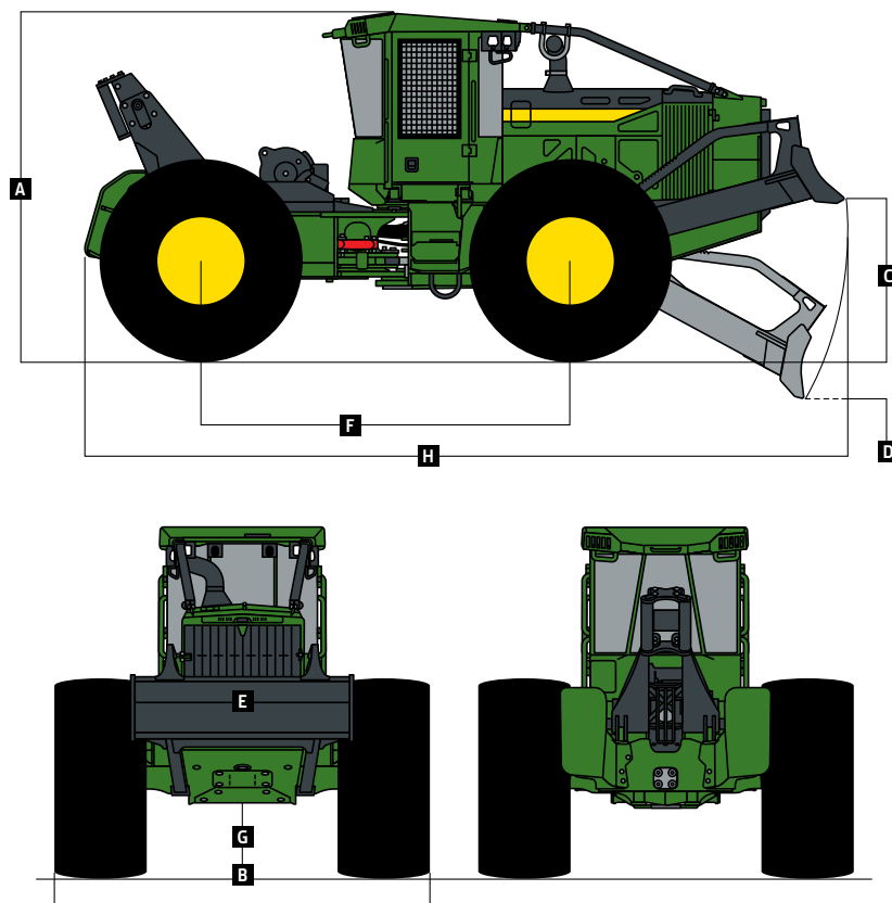
Skidder com Guincho 640L-III
